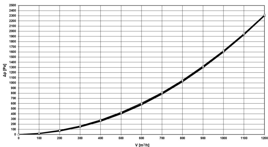
Sl. 21: Diagram izgube tlaka
